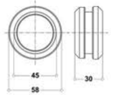
KSL-HN 50 Sliding Door Handle
