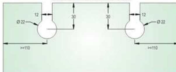
CUTOUT DETAILS OF SSL-44-A1
