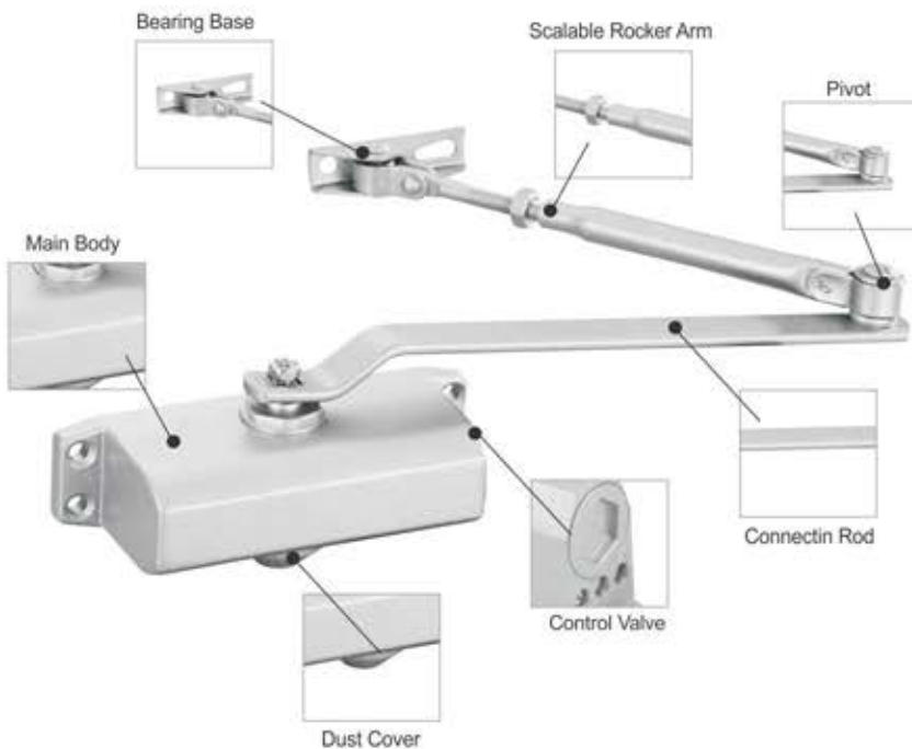
KDC-101 Door Closer (Sleek) Door Weight Capacity : 40-65 kg
